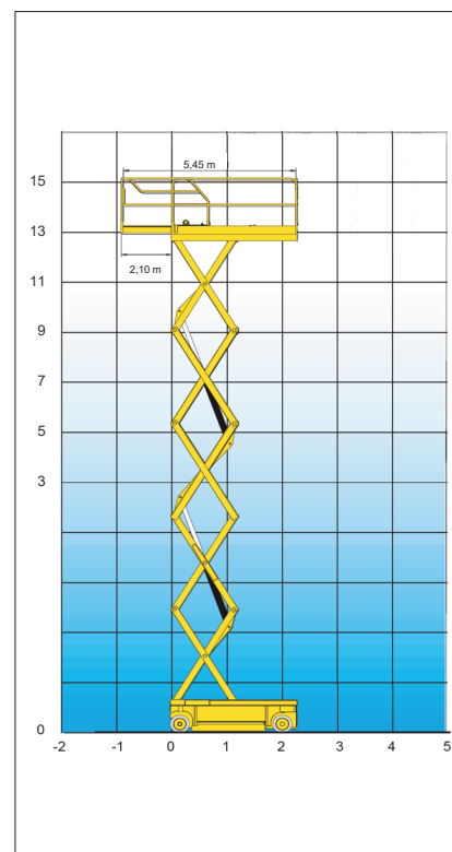
Abmessungen
